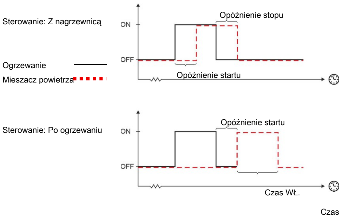
Rysunek 25: Sterownik z nagrzewnicą
