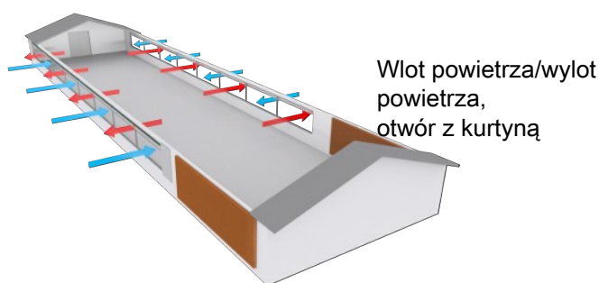
Rysunek 20: Przykład budynku inwentarskiego z wentylacją naturalną w połączeniu z wentylacją tunelową — wentylacja naturalna.
