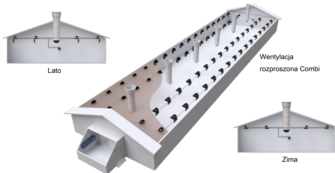
Rysunek 8: System wentylacji Combi-Diffuse to połączenie najlepszych cech dwóch systemów wentylacji: dyfuzyjnego i LPV.
