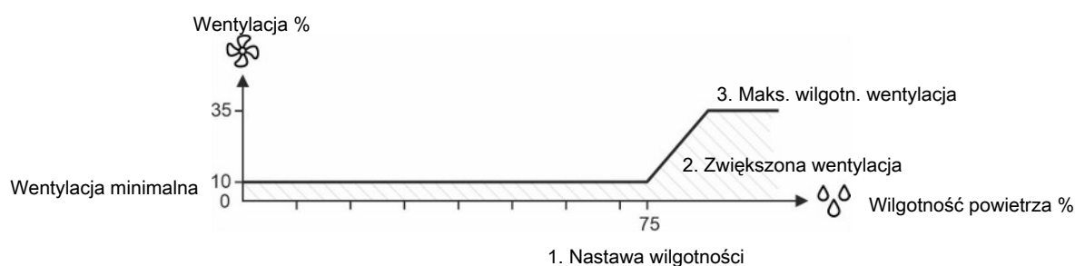
Rysunek 14: Regulowanie wilgotności przez wentylację: 1. Wilgotność powietrza przekracza nastawę wilgotności. 2. Sterownik zwiększa wentylację. 3. Zwiększenie wentylacji do regulowania wilgotności do wartości maksymalnej (35%).
