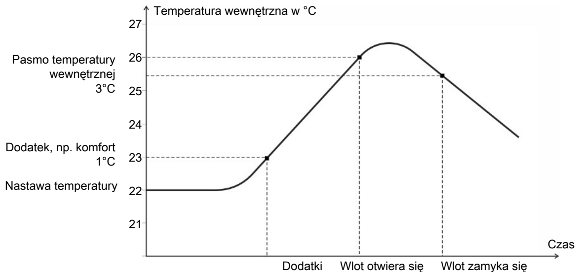
Rysunek 9: Wlot wentylacji łączonej — regulowana temperatura wewnętrzna
