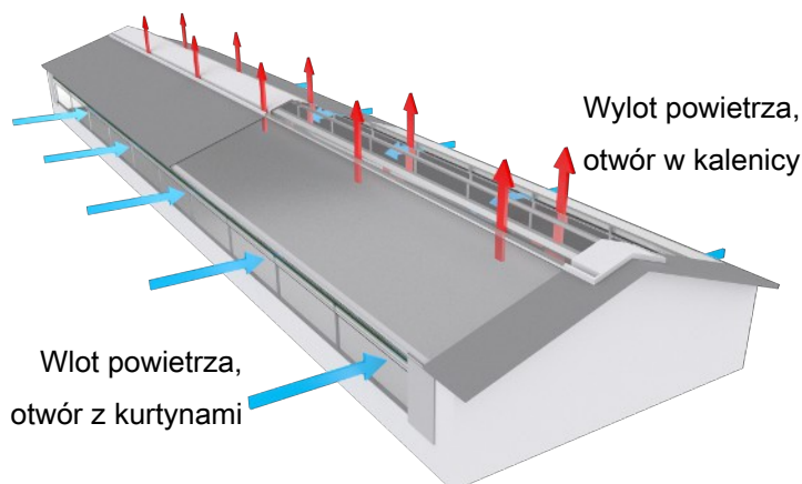
Rysunek 19: Przykładowo w budynku z czystą wentylacją naturalną z otworami z kurtynami po obu stronach i otworu w kalenicy.
