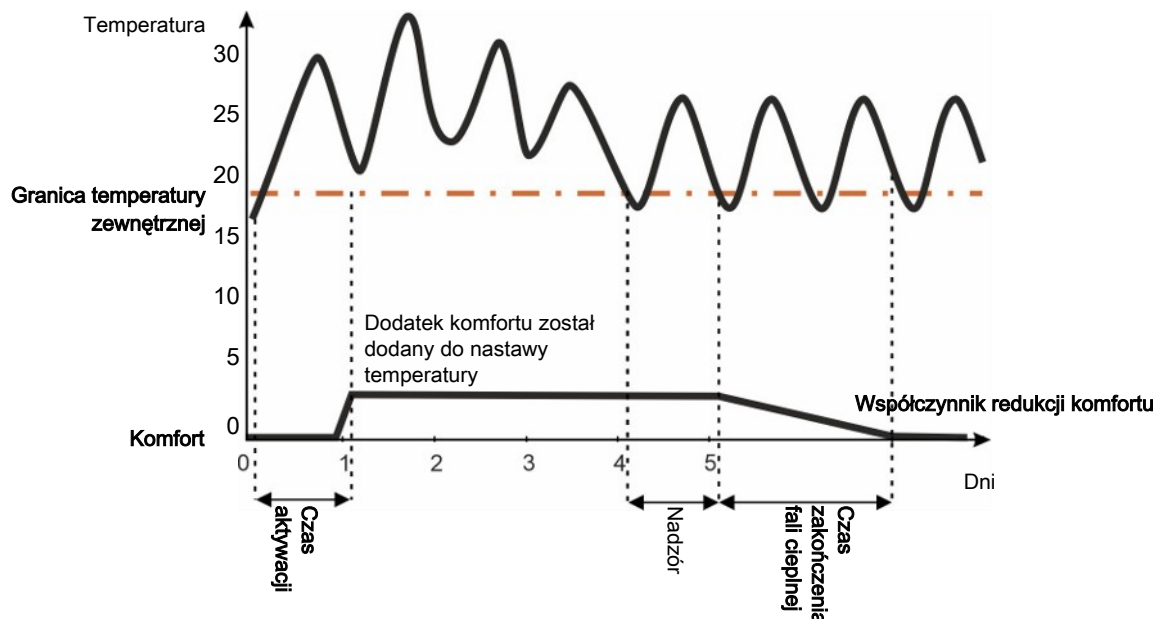
Rysunek 4: Komfort fali ciepłej
