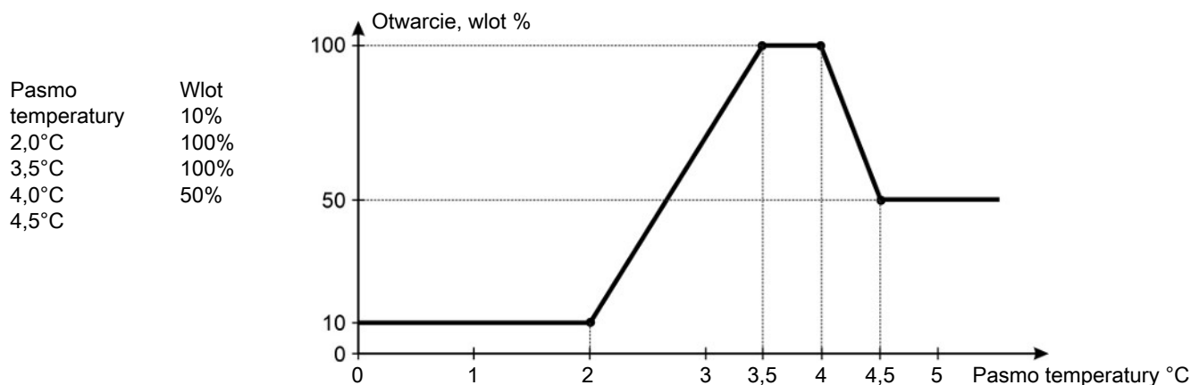
Rysunek 10: Wlot wentylacji łączonej — redukcja bezstopniowego otwierania przy wysokiej temperaturze zewnętrznej
