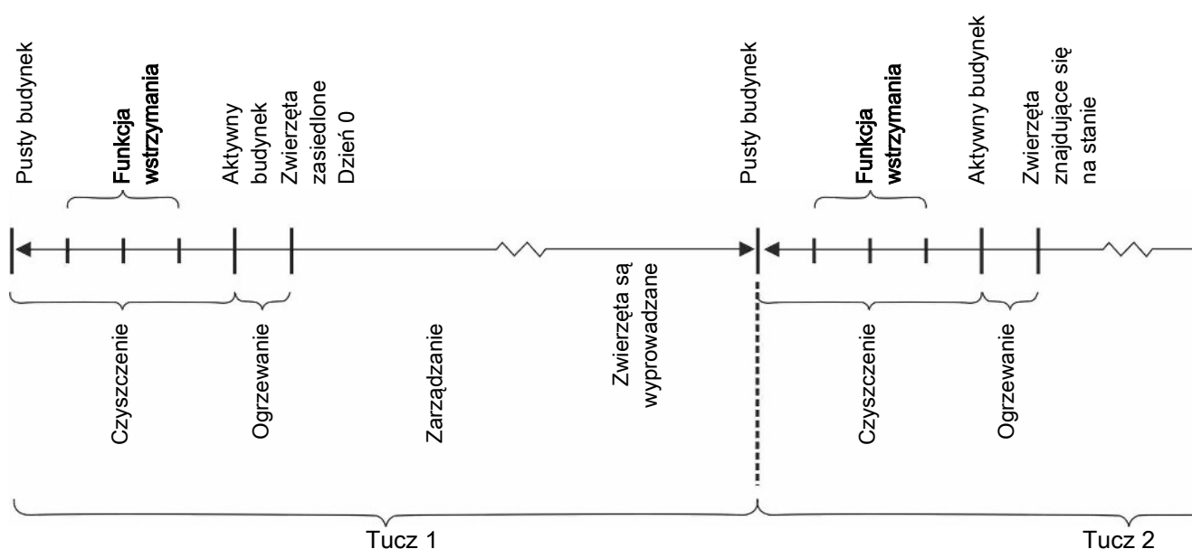
Rysunek 1: Przykład konfiguracji wstrzymania funkcji dla produkcji tuczu
